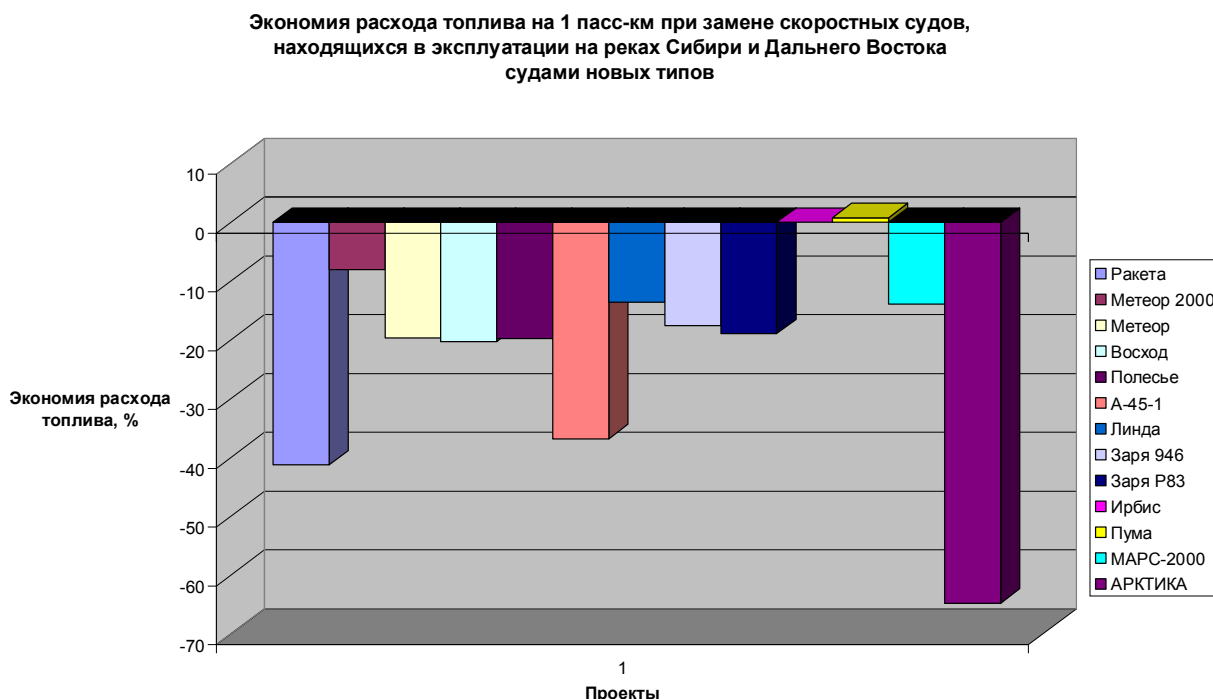
Рис. 1. Экономия расхода топлива на 1 пасс-км при замене скоростных судов, находящихся в эксплуатации на реках Сибири и Дальнего Востока, судами новых типов.
