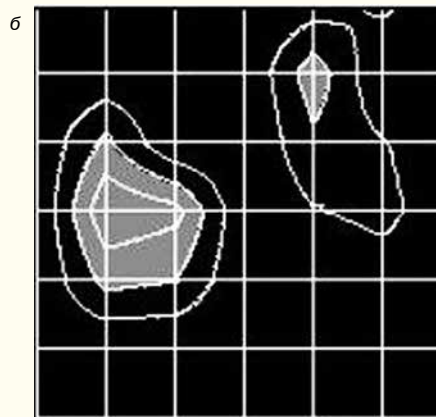
Рис. 6. Траектория движения ПЭП (а) и изображение дефектной зоны (б) при контроле методом свободных колебаний
